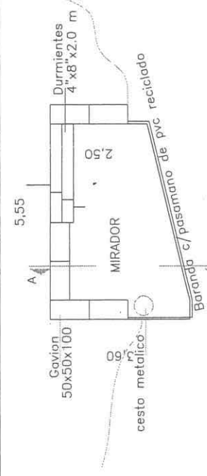
PLANTA
